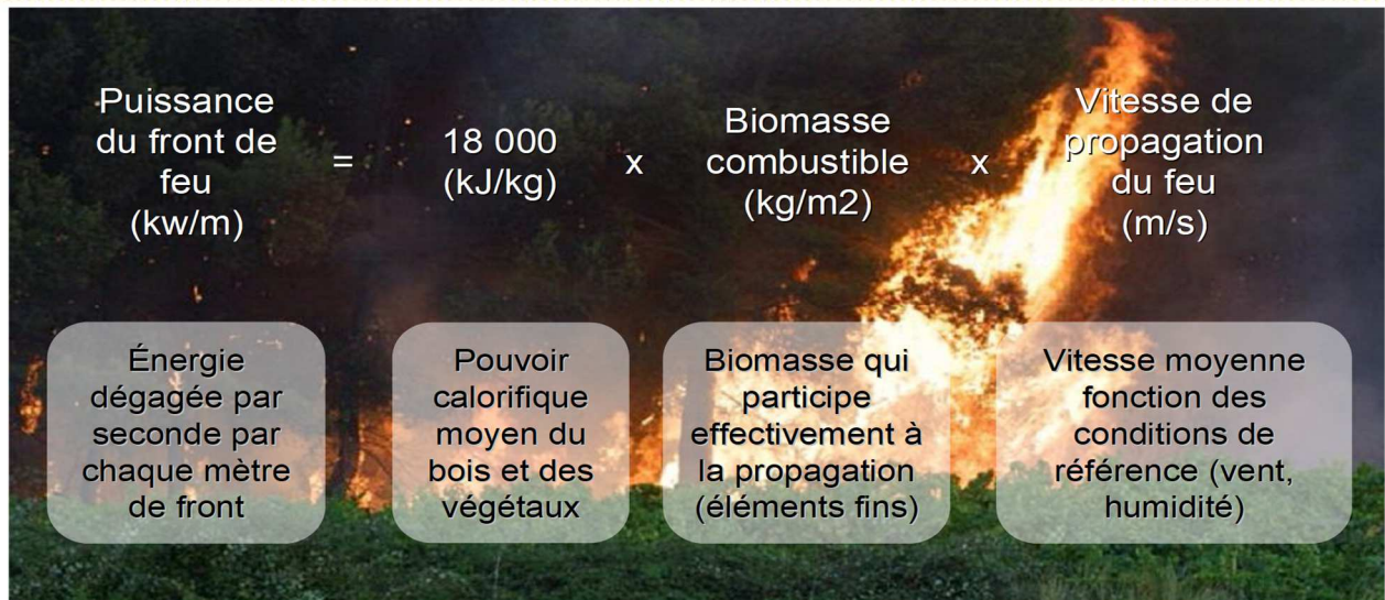
Figure 37 : formule de Byram
